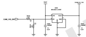
VCAM_IO_LDO
