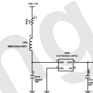
HALL IC
